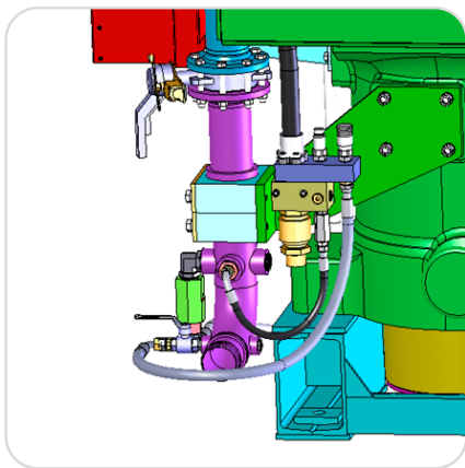
装配快速附件套件的3D渲染
